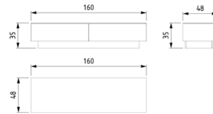
ÜNİTE ALT ÇİFTLİ BLOK
